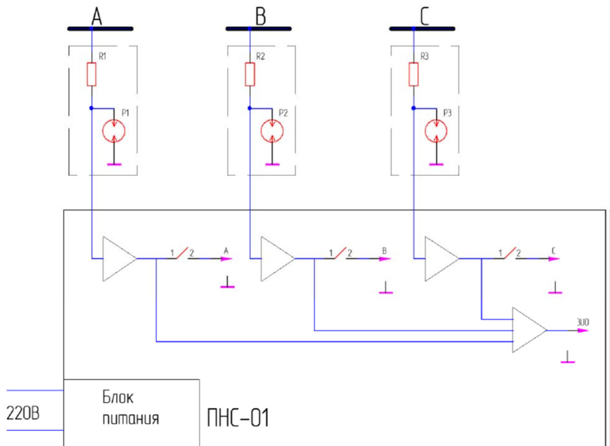
Структурная схема устройства ПНС-01 УХЛЗ.1
